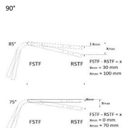
Pente d'assise en fonction du type de châssis
